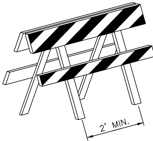
TYPE II BARRICADE
